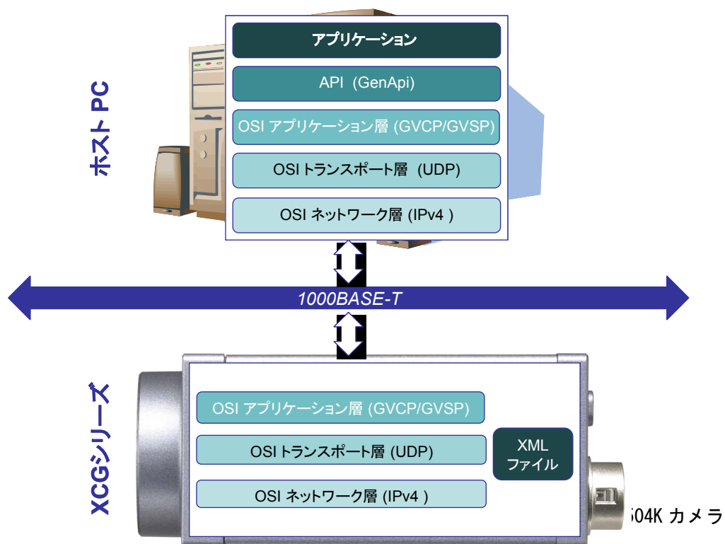
第 2 図 GigE Vision プロトコルスタック
