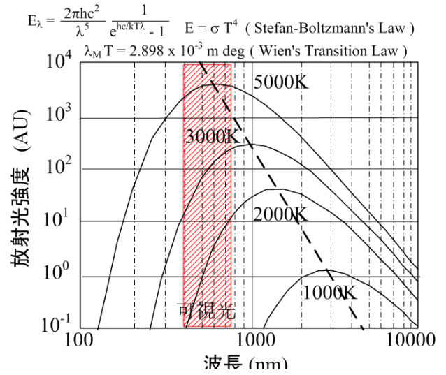
第 2 図 波長と熱(光)放射強度の関係
