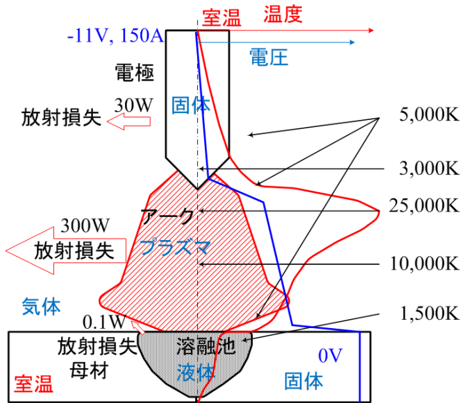
第 1 図 GTA 溶接の原理・概要
