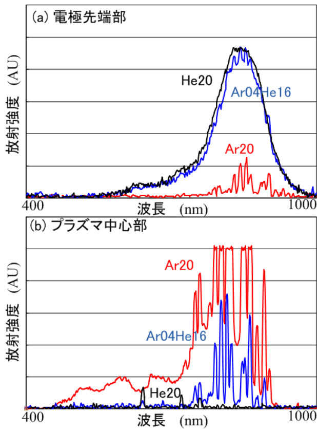
第 4 図 ガス種の違いによるスペクトル分布の変化
