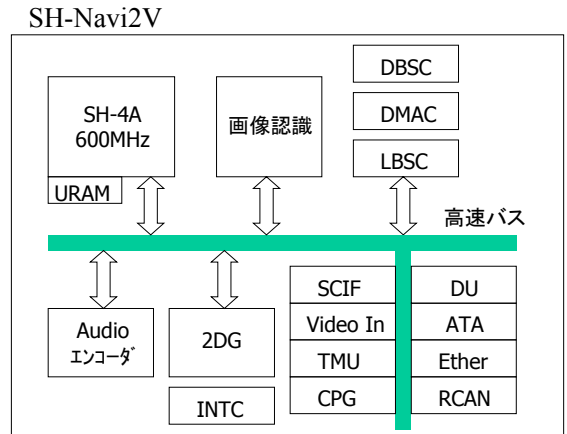
第 4 図 カーナビゲーション向け SoC の構成
