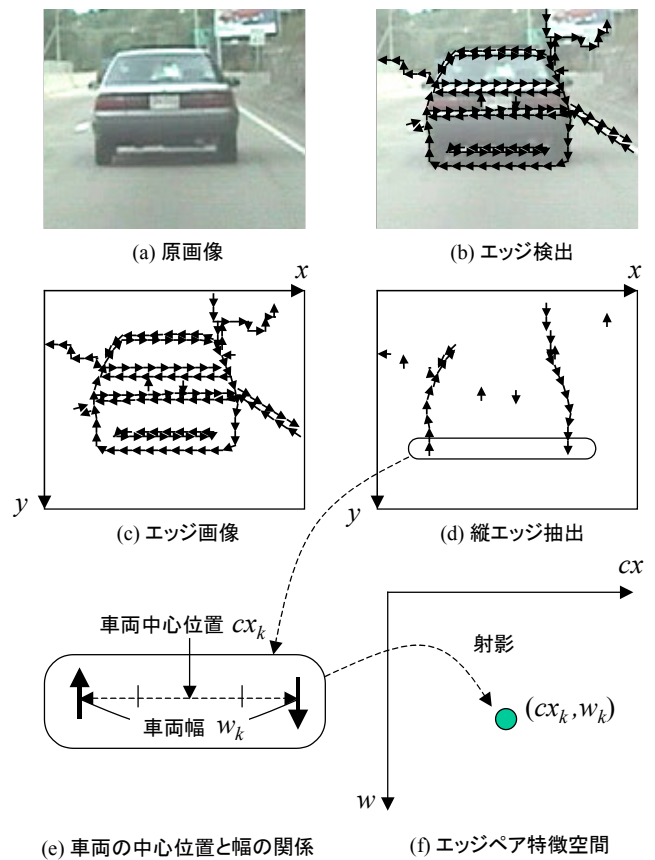
第 6 図 車両検地の処理フロー
