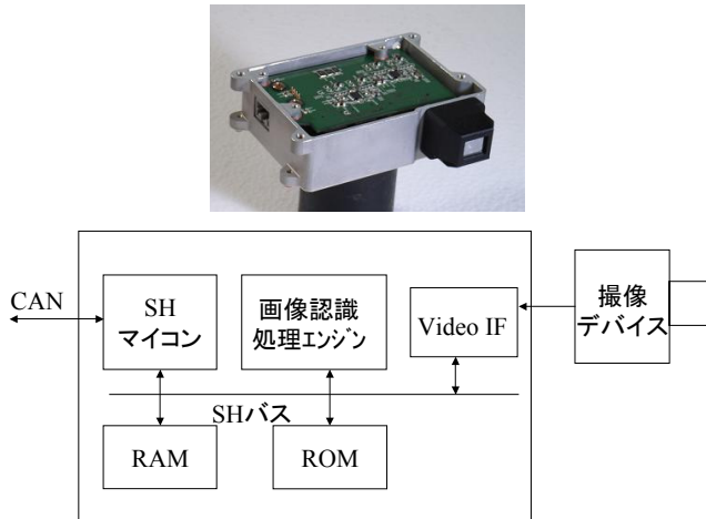
第 2 図 車載画像認識処理カメラの外観(上)と構成(下)
