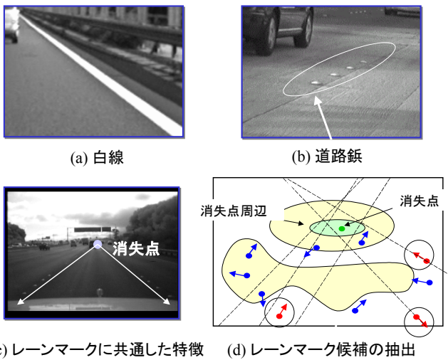
第 5 図 レーン認識対象(白線と道路鈺)
