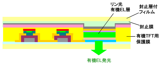
第 6 図 フレキシブル有機 TFT 駆動有機ディスプレイの構造
