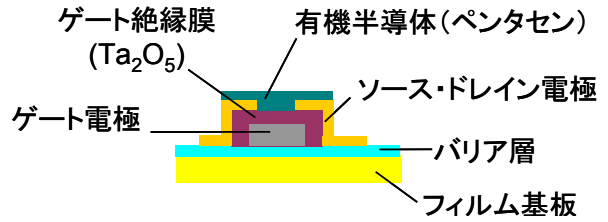
第 2 図 低電圧動作有機 TFT の構造
