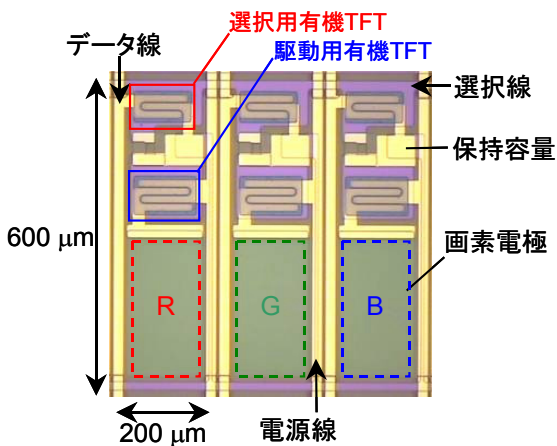
第 4 図 画素表面の顕微鏡写真
