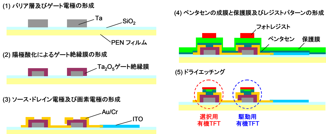
第 3 図 フレキシブル有機 TFT アレイ作成プロセス
