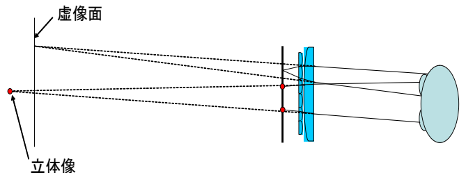
第 2 図 粗インテグラルイメージングにおける虚像光学系
