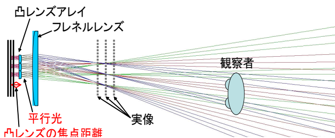
第 4 図 粗インテグラルボリュームイメージングの光学系
