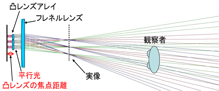
第 1 図 粗インテグラルイメージングにおける実像光学系
