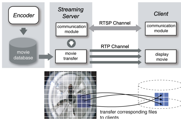
第 7 図 サーバ・クライアント通信の概略
