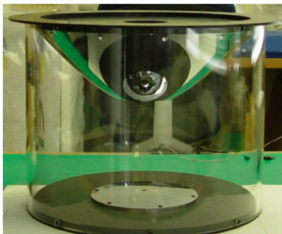
第 4 図 2 枚反射系全方位ミラー
