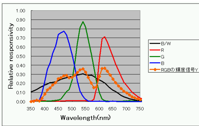
第 6 図 CCD の感度特性
