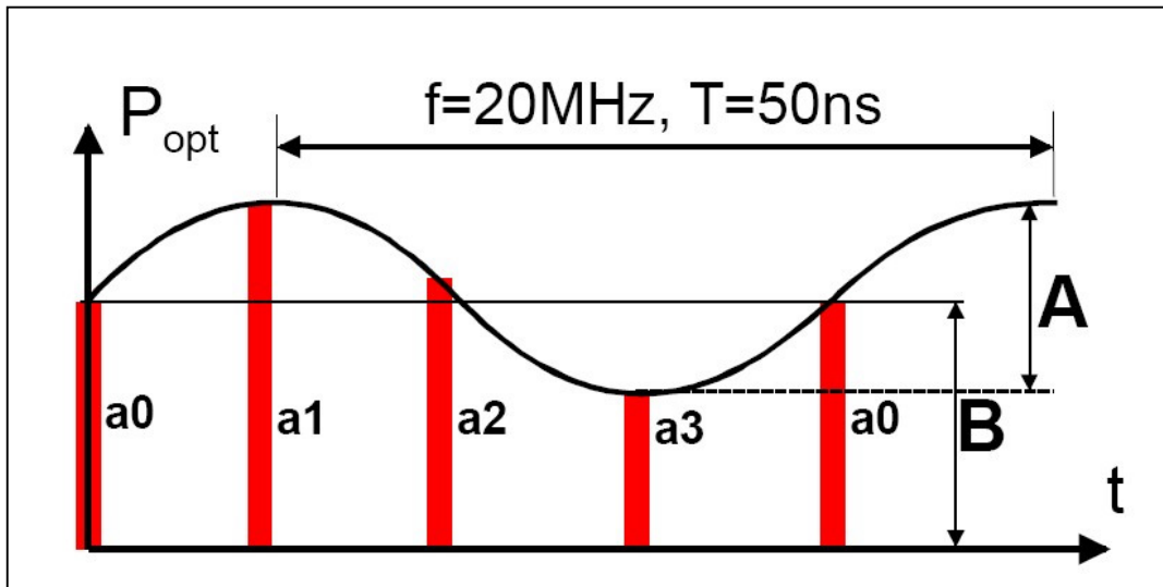
第 2 図 4 点サンプリングを用いた TOF3 次元レンジファインダの原理図
