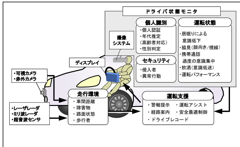
第 1 図 予防安全のための運転支援システム
