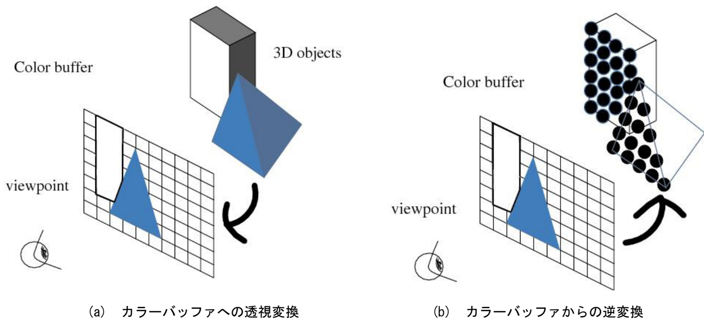
第 1 図 カラーバッファへの透視変換と逆変換
