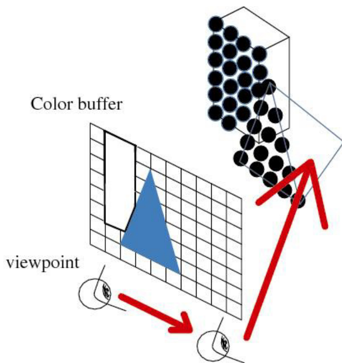
第 3 図 視点移動による隠れ面の欠陥
