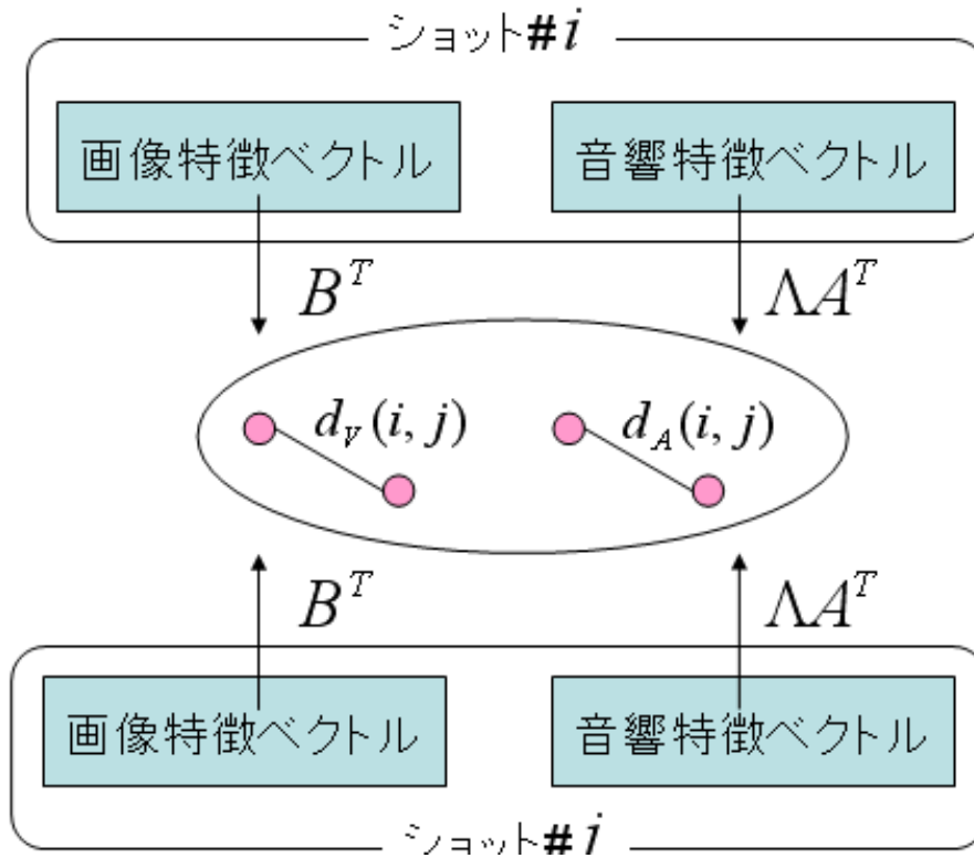
第 1 図 画像、音響特徴の同一空間への写像
