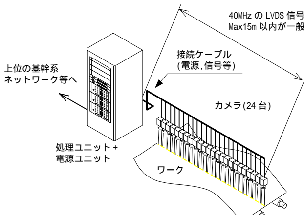
第 1 図 一般的な他カメラ検査システムの例
