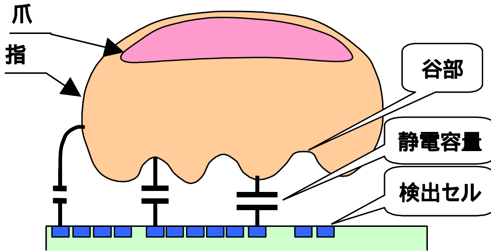
第 1 図 静電容量式の指紋センサ
