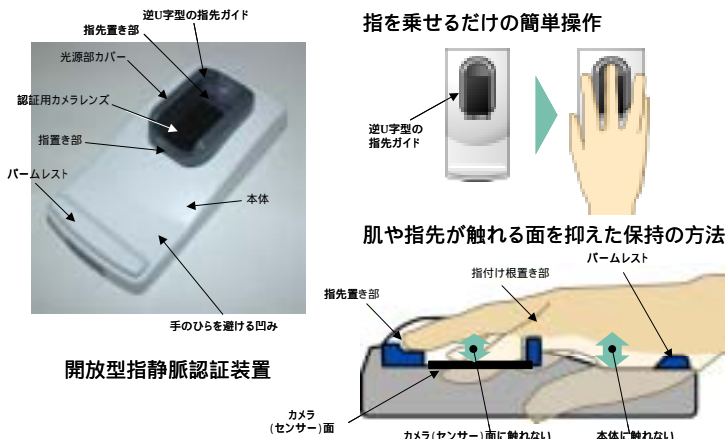
第3図 開放型指静脈認証装置
