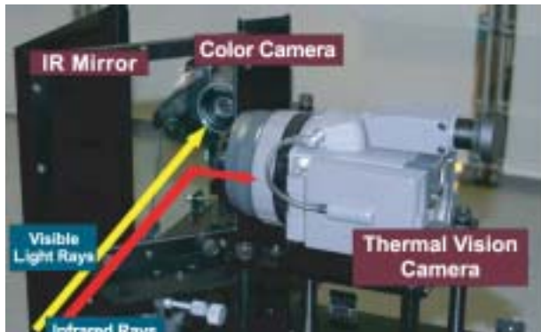
第 1 図 thermo-key の構成
