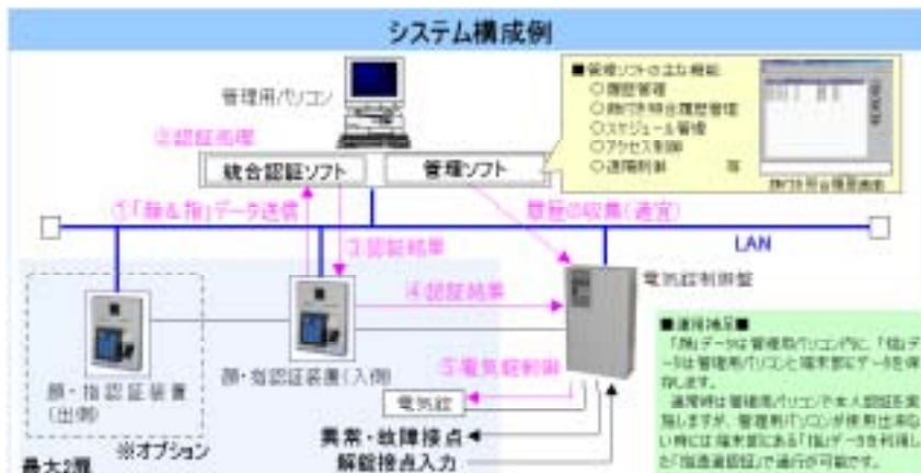
第 3 図 システム構成：出入管理用の顔・指認証装置のシステム構成例
