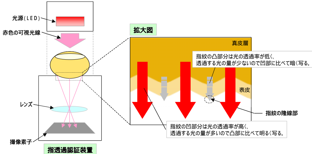
第 1 図 指透過認証装置：指内部の光透過率の変化により，指の内部組織を光学的に検出する
