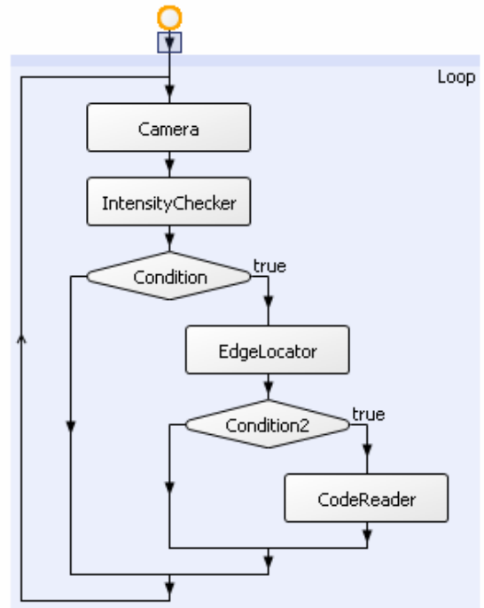
第 2 図 DA のフローチャート
