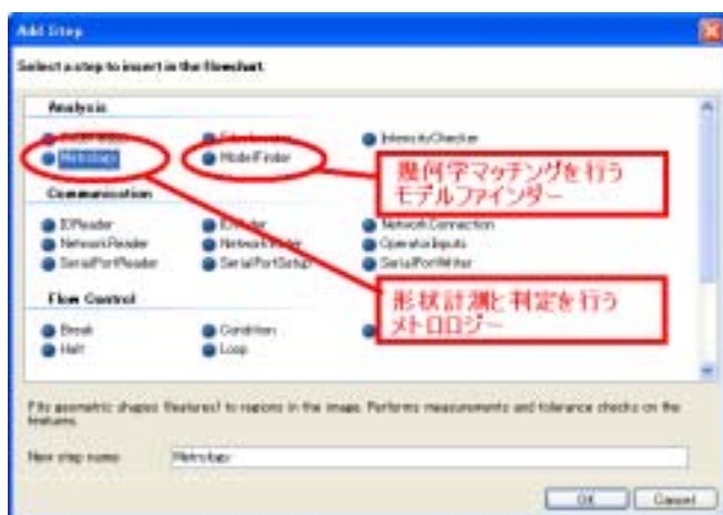
第 5 図 DA機能リスト
