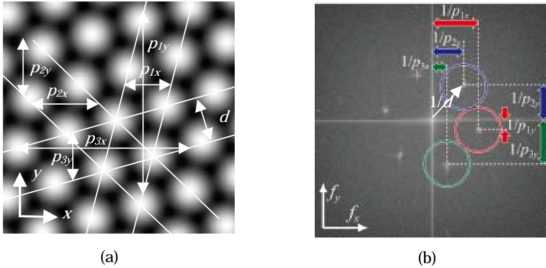
第 3 図 六方格子とそのスペクトル
