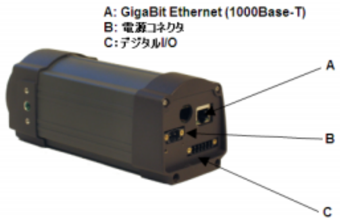
写真 7 A320G 背面パネル
