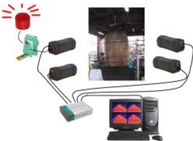
写真 6 A320 システム構築例
