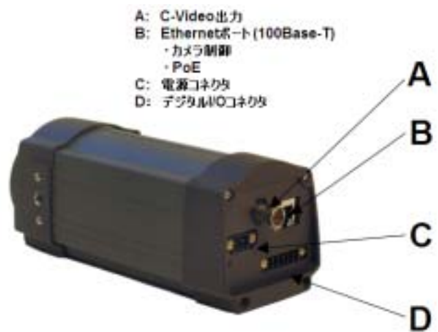
写真 5 A320 背面パネル
