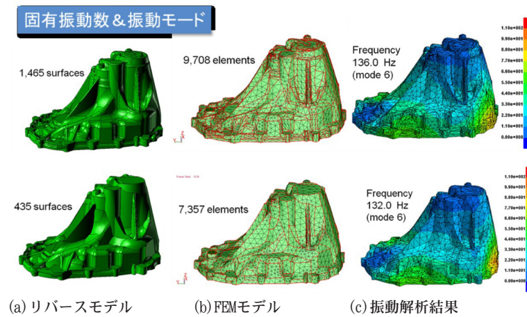
第 4 図 解析事例
