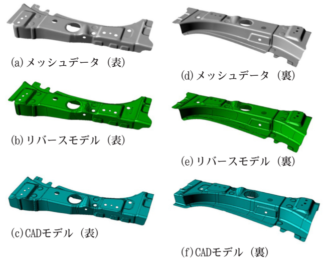
第 3 図 リバースモデルとCADモデルの比較
