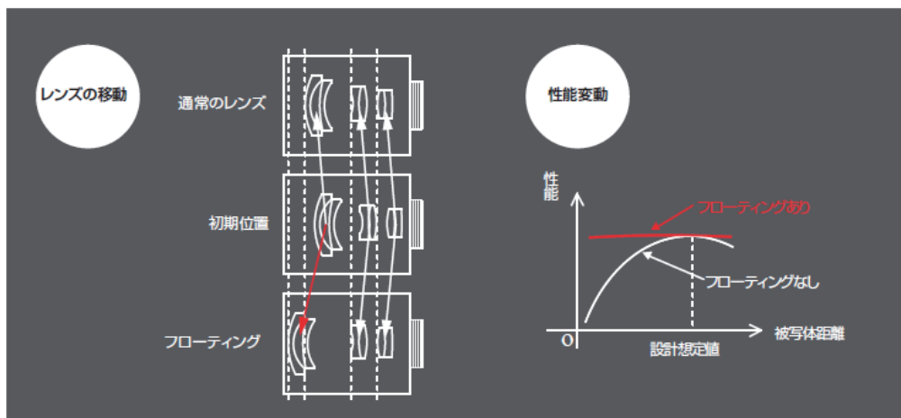
第 2 図 フローティング構造
