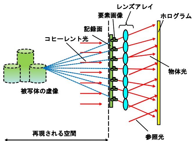
第2図 ホロコーダホログラムの記録
