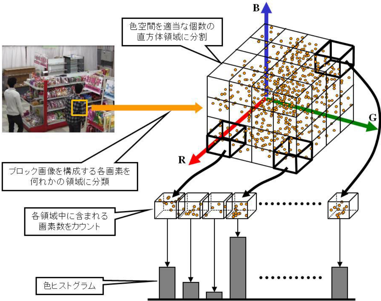
第 8 図 色ヒストグラム特徴量
