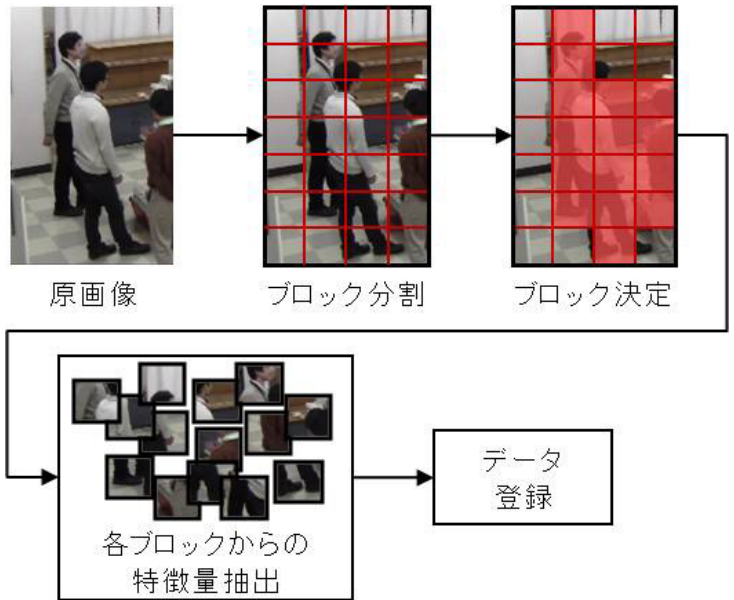
第2図 ブロック画像を対象としたデータ登録処理
