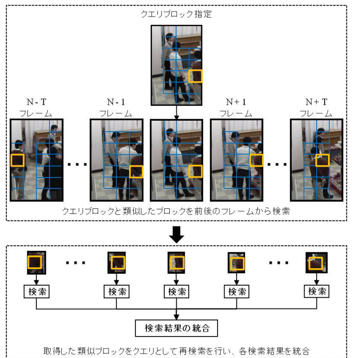
第4図 複数クエリ生成方式を用いた検索処理
