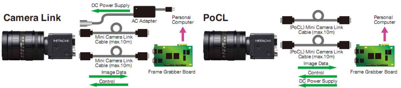
第1図 ダブルカメラリンクインターフェース接続図
