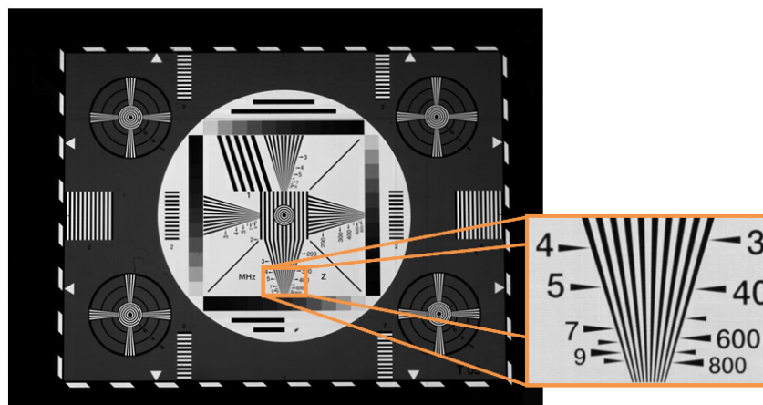
第5図 CMV12000のテスト画像
