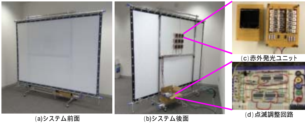
第5図 盗撮防止システムの外観
