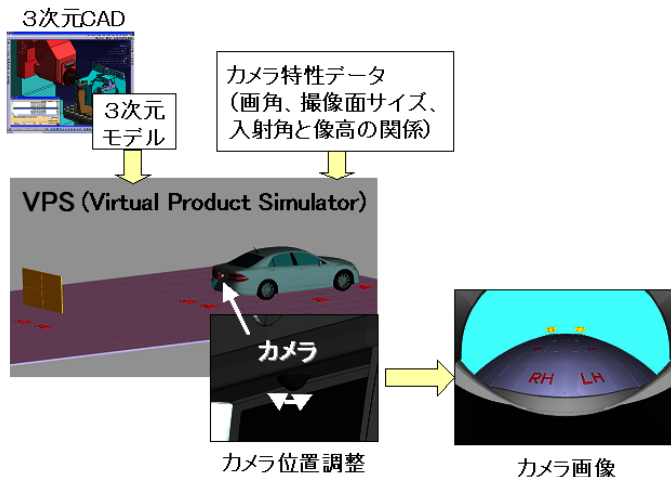
第3図 カメラ配置設計システム
