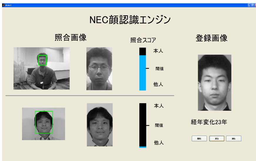
第8図 照合結果例
