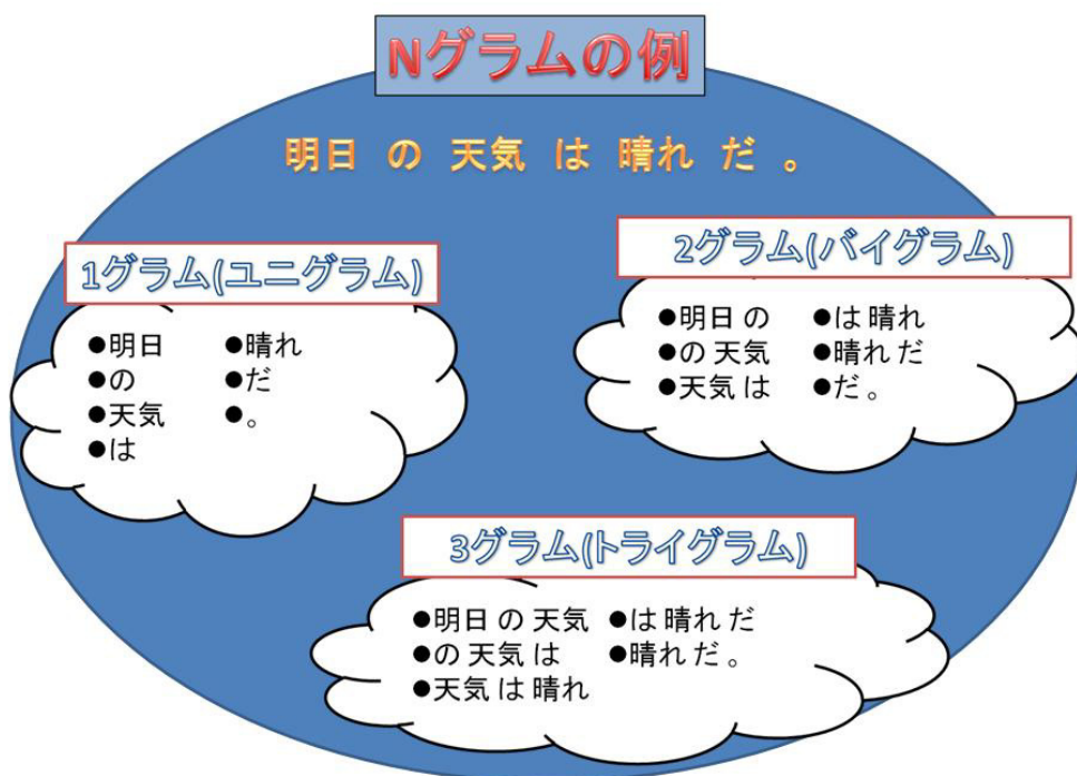
第2図 Nグラムの例
