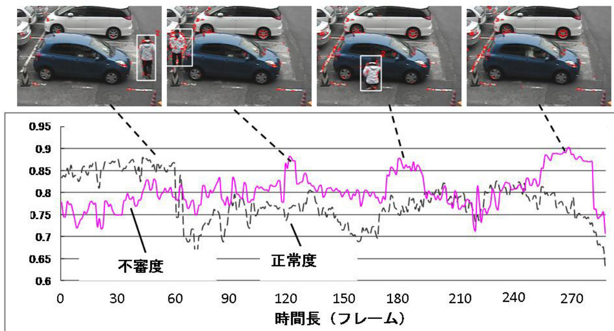
第3図 実験結果例(部分空間法+AdaBoostによるデータ選択)
