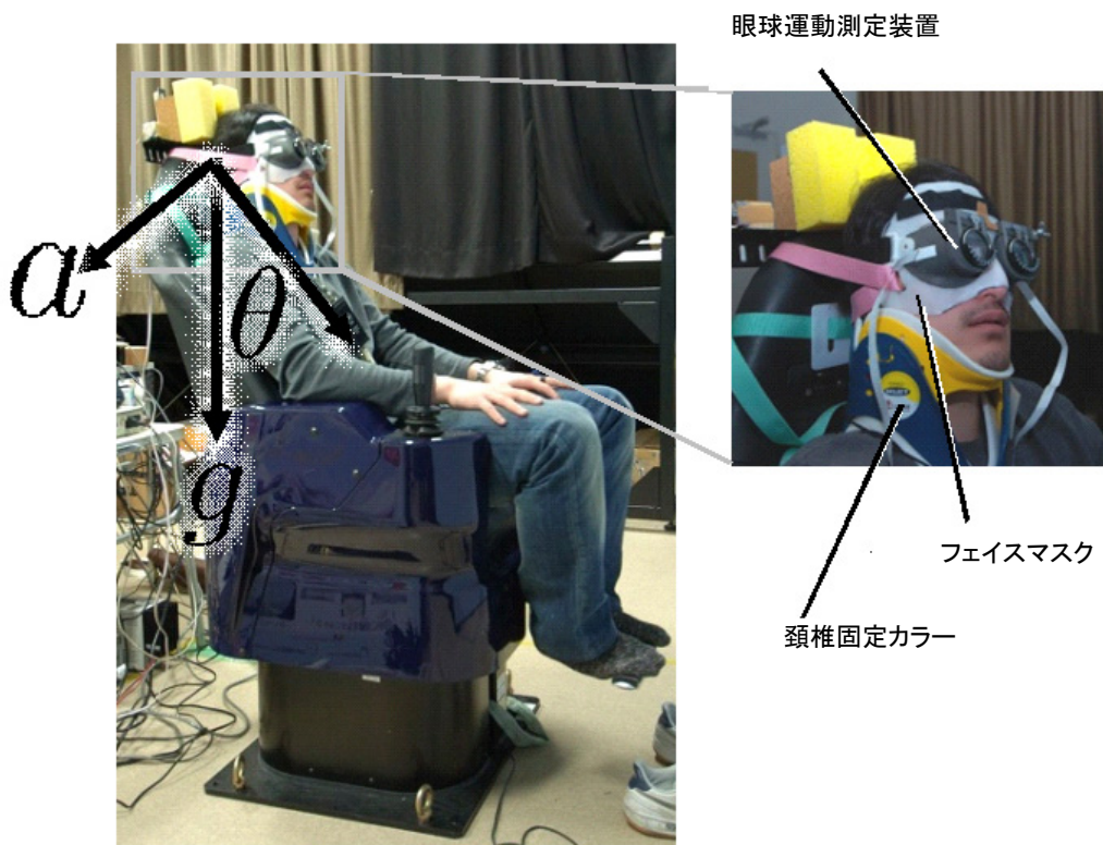
第2図 モーションチェアと眼球運動測定装置
