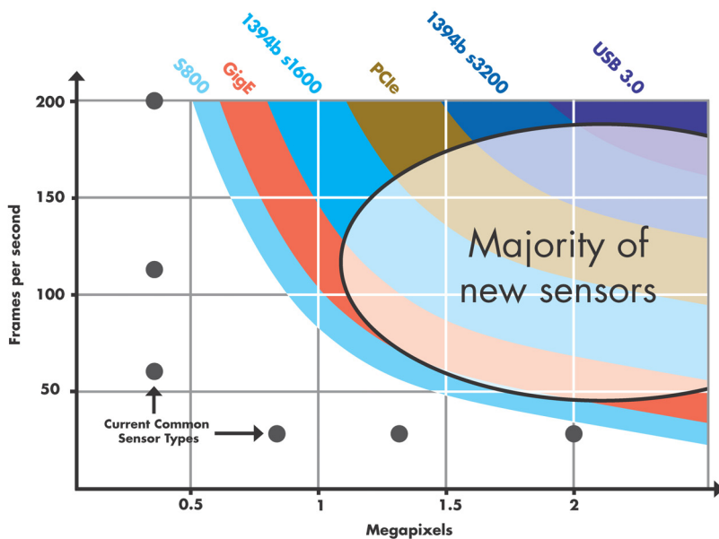
第 4 図 新センサーには新しいインターフェースが必需
