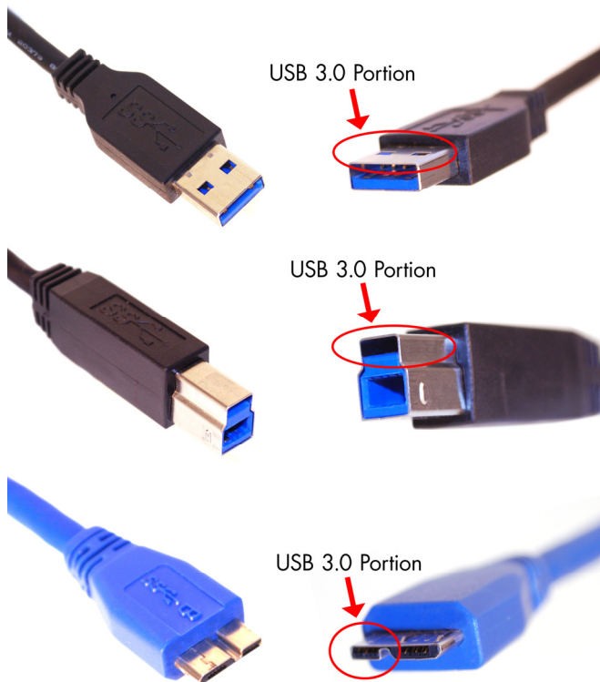
第 1 図 CUSB3.0 はコネクタ及びケーブルの互換性重視の設計
