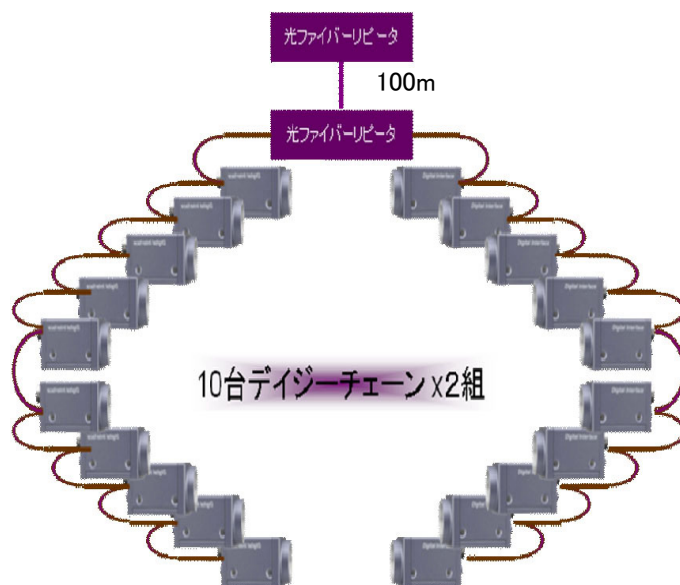
第5図 システム事例
