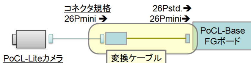
第8図 Lite～Base 変換ケーブル
