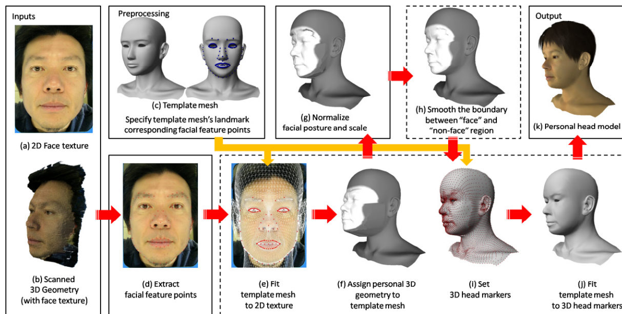
第1図 提案手法の概要
