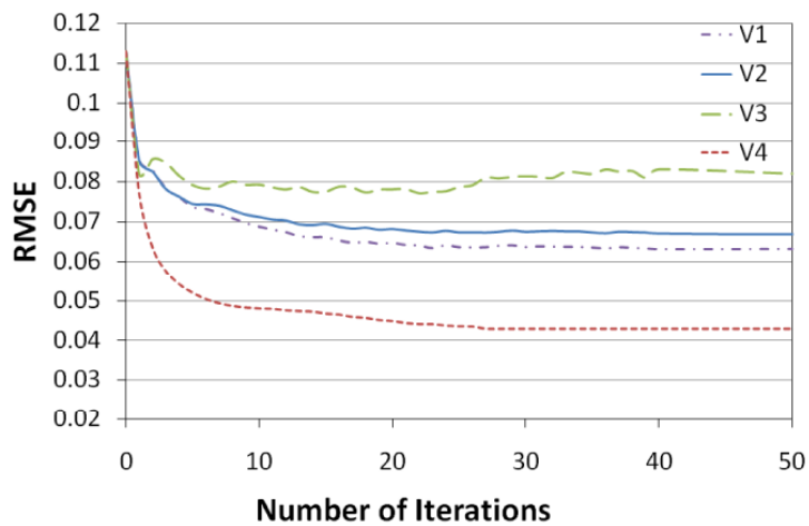
第5図 V1～V4 の最適化反復回数毎の RMSE
