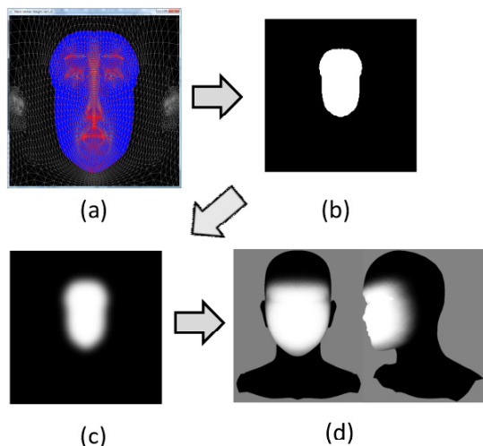
第2図 顔形状重要度マップの作成
