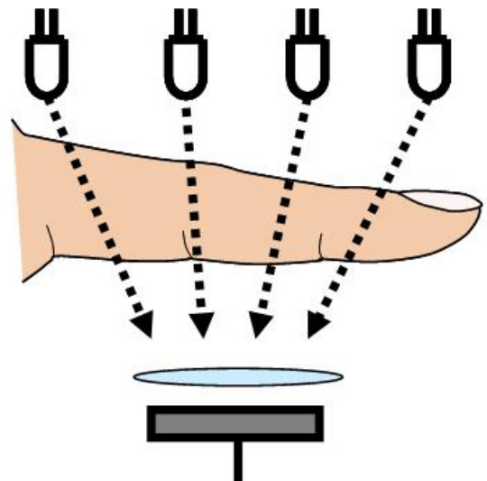
(b)透過光センシング
