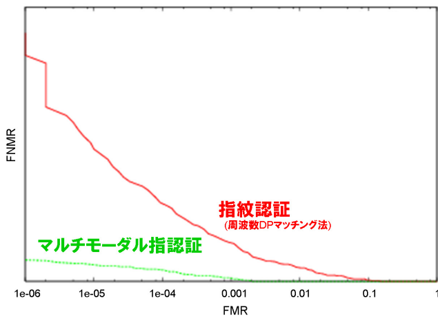
第 5 図 ROC 曲線による比較
