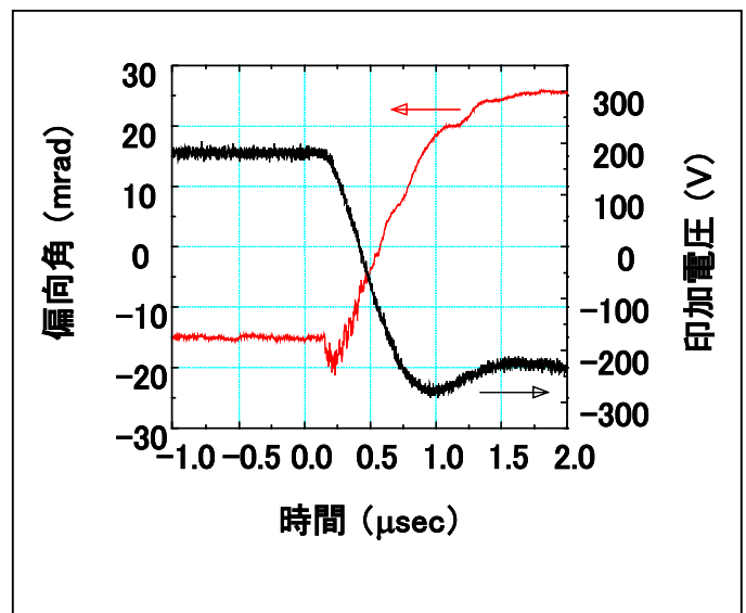
第3図 KTNスキャナーの高速応答特性
