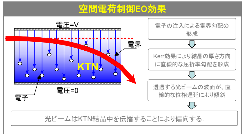
第1図 KTN結晶中の空間電荷制御EO効果
