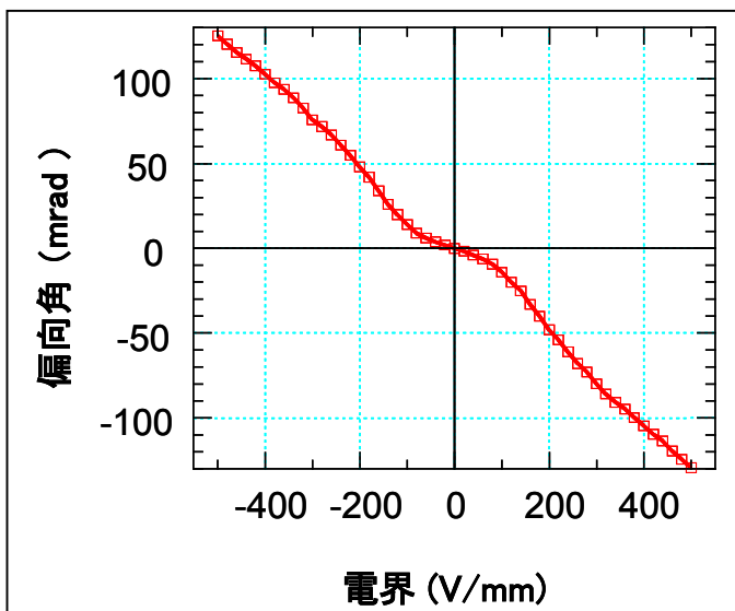
第2図 偏向角の電界依存性
