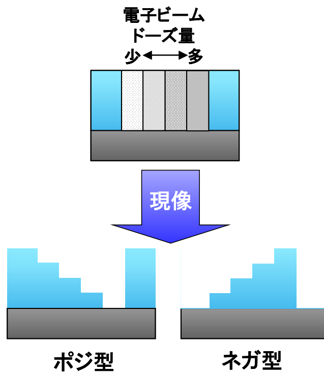
第 3 図 電子ビーム露光法において、ドーズ量を変えたときの高さの変化
