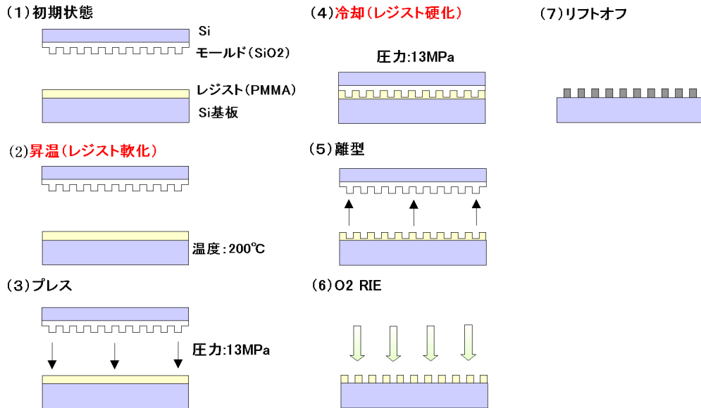
第 1 図 ナノインプリントリソグラフィーの工程図
