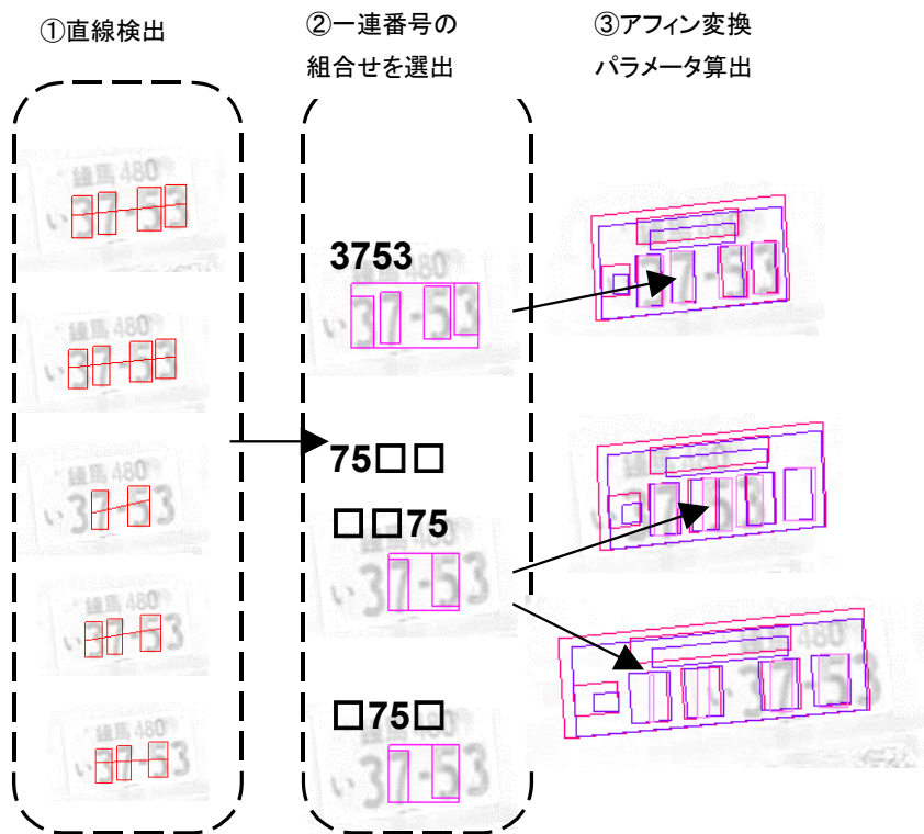
第 10 図 ナンバープレート認識アルゴリズムの概要 画像中から直線状に並ぶ数字候補を抽出し (①)、一連番号のどの桁に相当するかを評価 (②)、アフィン変換パラメータを算出する (③)。
