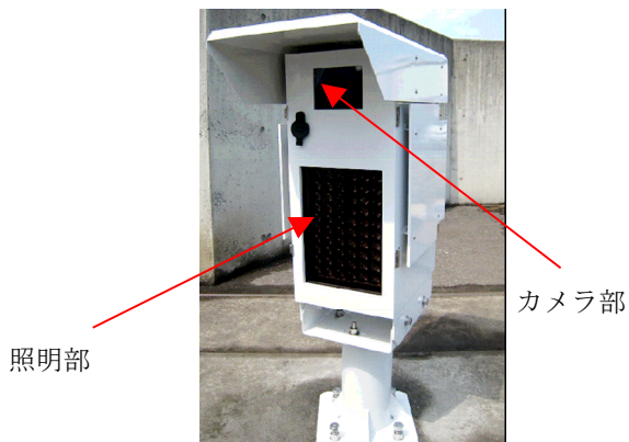
第 1 図 撮像部の外観 白黒メガピクセルカメラおよび高輝度赤外線照明で構成されている
