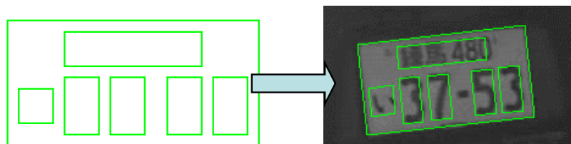
第 9 図 テンプレートをナンバープレート画像に当てはめた例 ナンバープレートが正しく認識された場合には、用意したテンプレートが画像中のナンバープレートの適切な位置に重なる。
