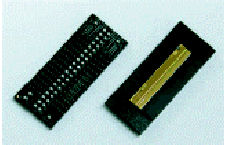
第2図 MBF310 指紋センサ
