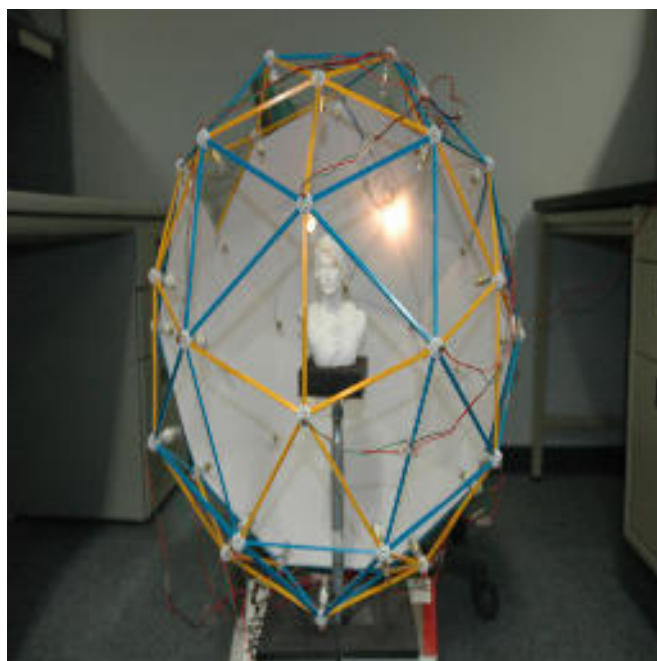
第 4 図 実験装置
