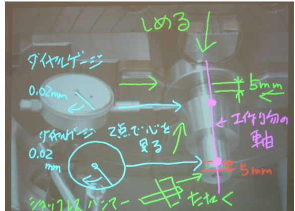
第2図 映像装置を使用した2点心出し作業の説明
