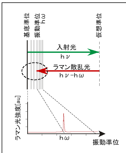
第 3 図 ラマン散乱光とラマンスペクトル
