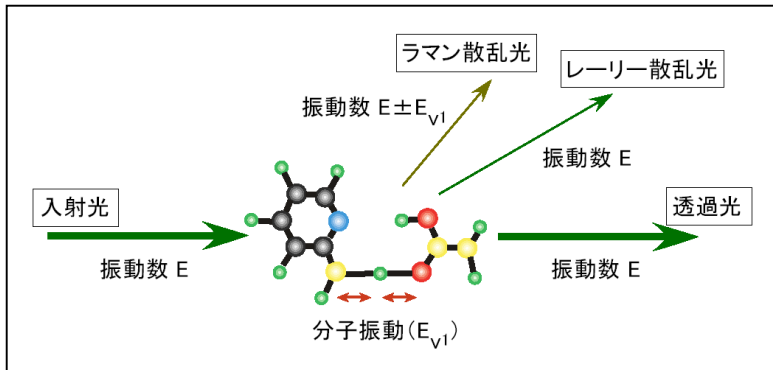
第 1 図 ラマン散乱光の模式図
