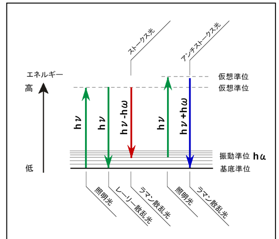
第 2 図 ラマン散乱とエネルギー準位図
