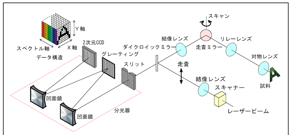
第 5 図 実際のラマン顕微鏡の原理
