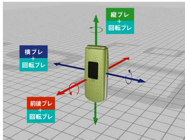
第 5 図 カメラの 6 自由度の動き
