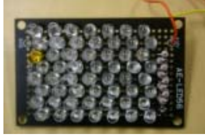
第 2 図 赤外線 LED を用いた 操作光源
