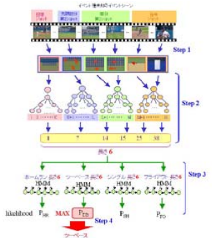
第 6 図 イベント識別処理の流れ
