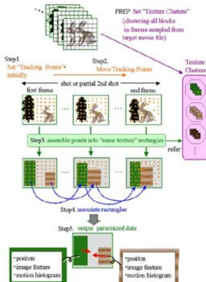
第 3 図 区間映像のパターン化処理
