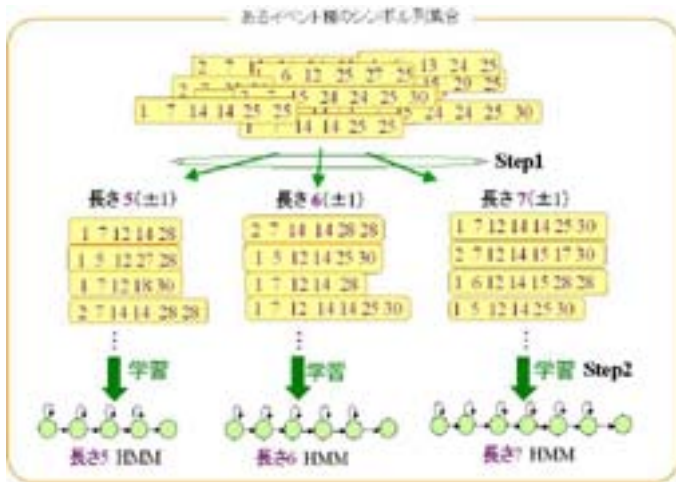
第 4 図 HMM の構築
