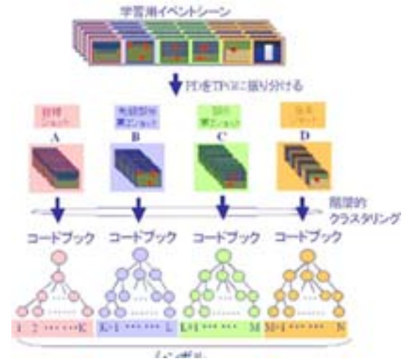
第 5 図 コードブック作成の全体の流れ
