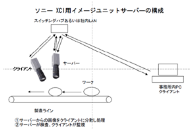
第 1 図 イメージユニットサーバー + XCI-V3 構成図
