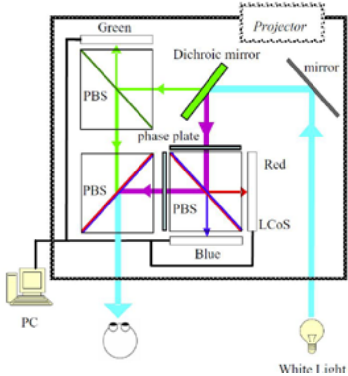
第 3 図 再生光学系
