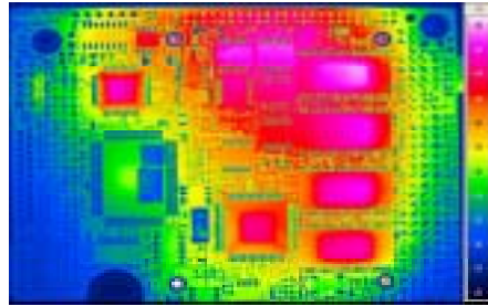
第1図 プリント基板の熱分布
