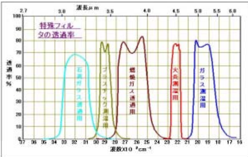
第5図 特殊フィルタの透過率
