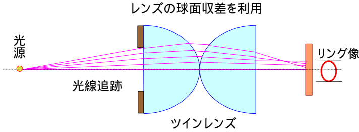
第 1 図 ツインレンズによるリング像の形成
