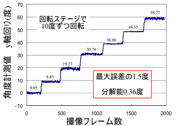
第7図 .51mmカードの角度計測 y軸周り@4m
