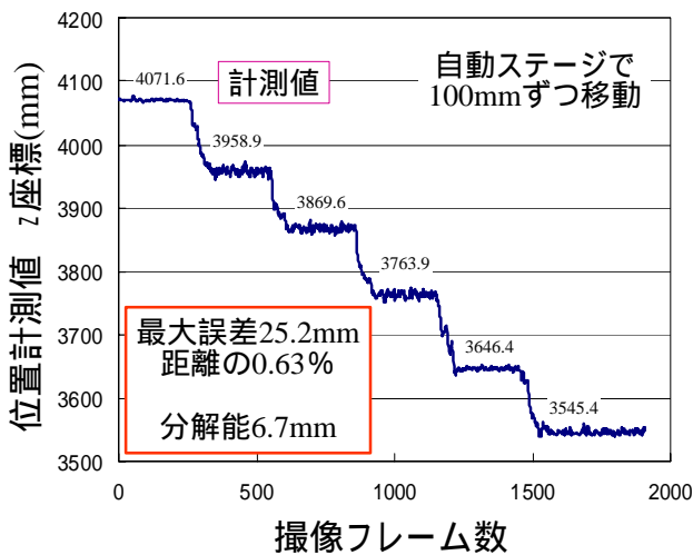
第6図 51mmカードの位置計測 z軸方向@4m
