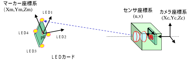
第2図 LEDカードの位置と角度の計測
